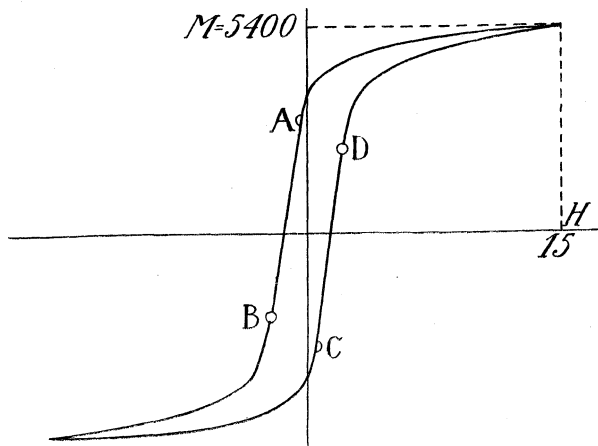
Fig. 4 (ijzer).
