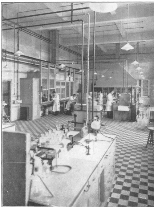
Fig. 12. Chemisch Laboratorium.
