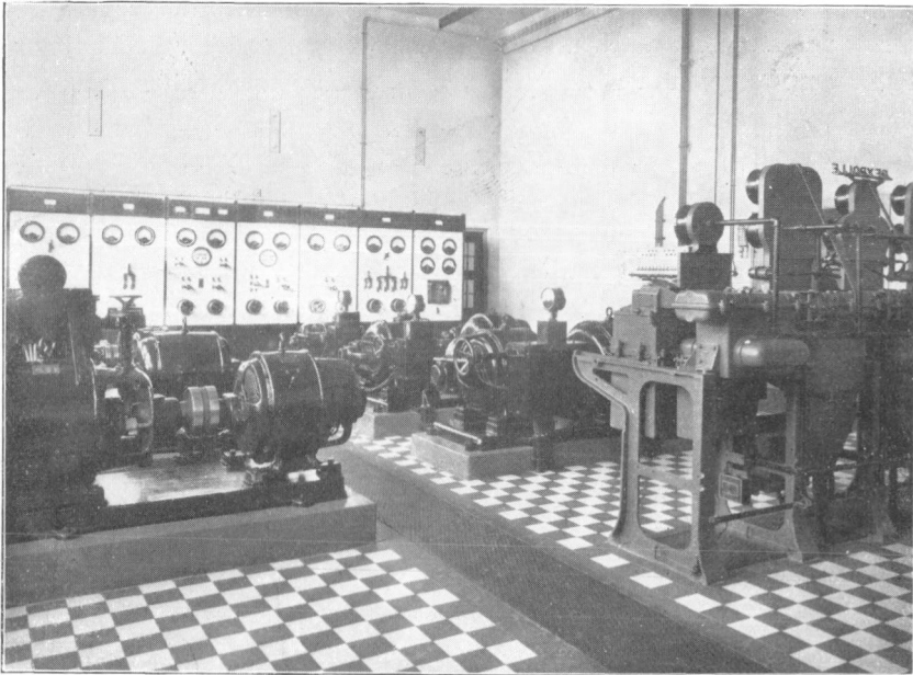
Fig. 4. Het dynamo-lokaal.
