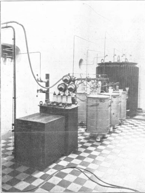
Fig. 13. Gelijkrichterinstallatie.
